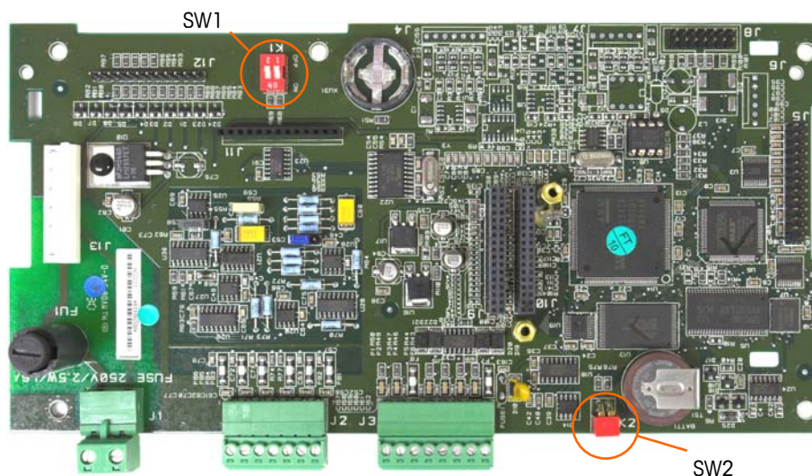
Figura 2-49: Interruptores del PCB principal
