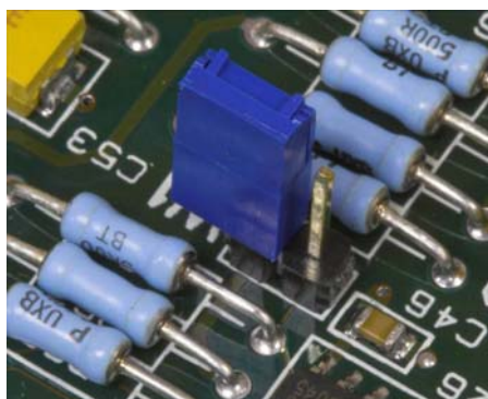
Figura 2-53: Selección de la conexión en puente de milivoltios
