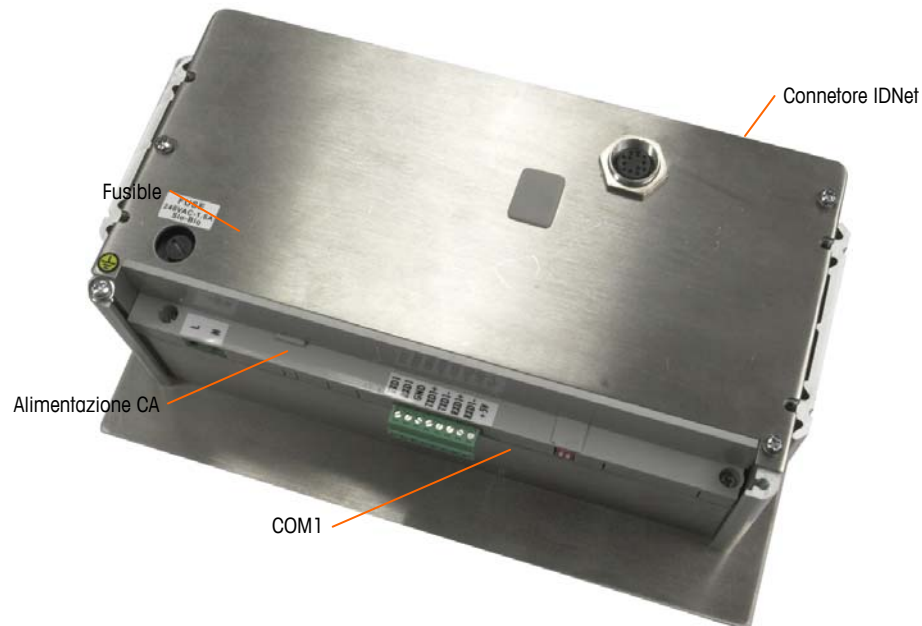
Figura 2-16: Versione IDNet in armadietto con montaggio a pannello
