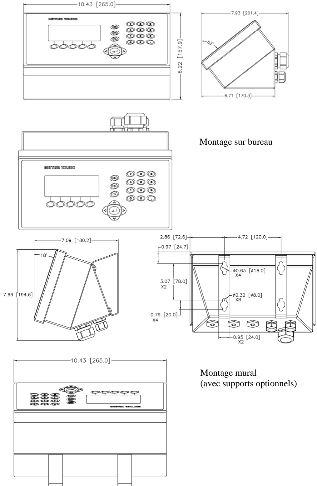
Figure 1-4 : Dimensions du terminal IND560 pour l'enceinte de montage mural/sur bureau/pour environnement hostile
