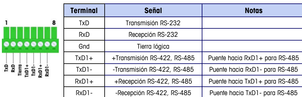
Figura 2-21: Señales del puerto COM1
