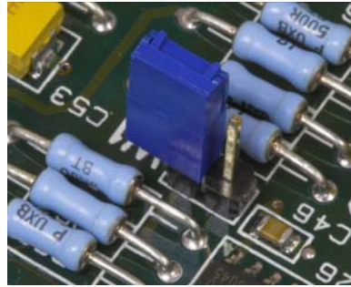
Figura 2-53: Selezione ponticello millivolt W1
