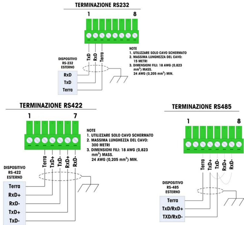
Figura 2-22: Esempi di collegamenti
