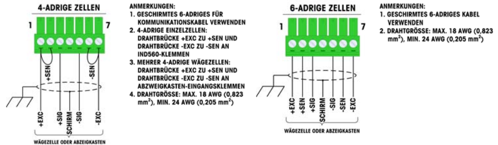
Abbildung 2-17: Wägezellenabschluss
