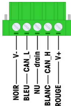
Figure 2-40: Câblage du connecteur DeviceNet
