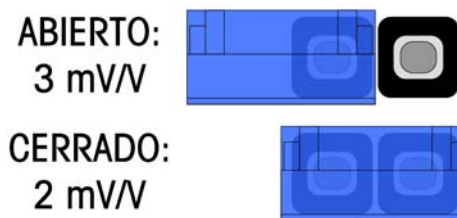
Figura 2-53: Selección de la conexión en puente de milivoltios
