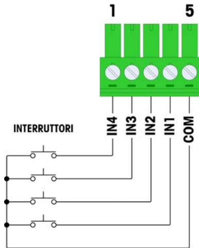
Figura 2-33: Connessioni dell'ingresso attivo
