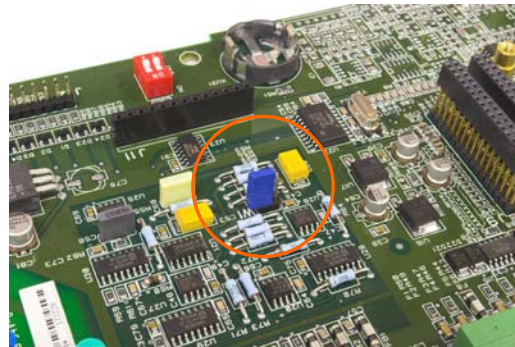
Abbildung 2-51: Lage der W1-Millivolt-Drahtbrücke, Hauptplatine ohne Abdeckung
