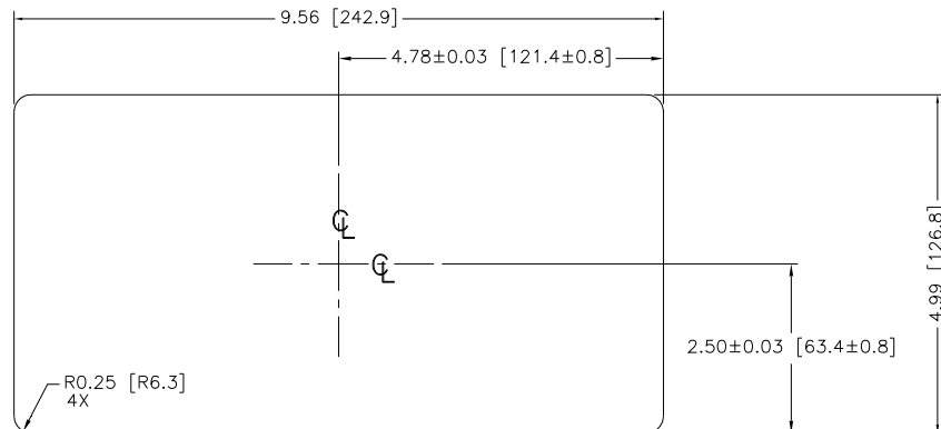
Figure 1-3 : Dimensions de découpe du montage sur tableau de l'IND560
