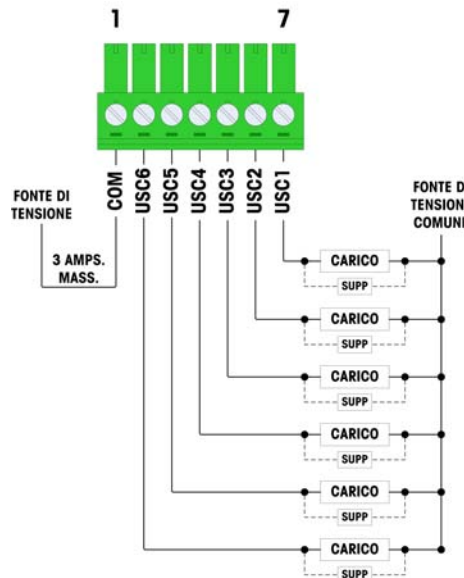
Figura 2-35: Uscite del relè
