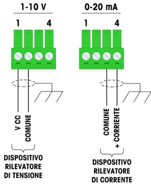
Figura 2-26: Terminazione uscita analogica
