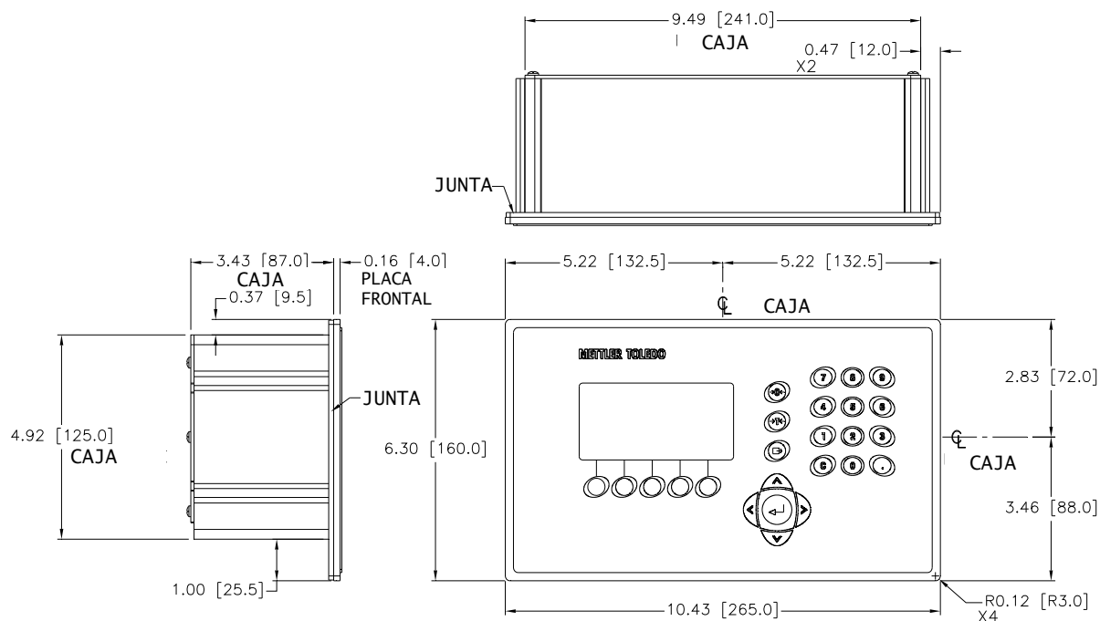
Figura 1-2: Dimensiones de la caja tipo montaje en panel del IND560
