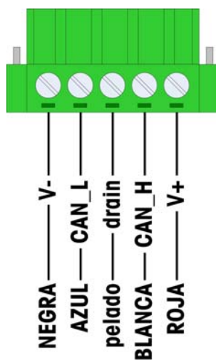
Figura 2-40: Cableado del conector de DeviceNet
