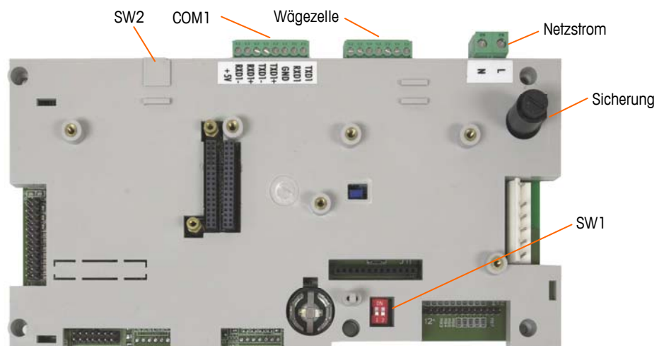
Abbildung 2-15: Analog-Hauptplatine in Gehäuse für raue Umgebungen
