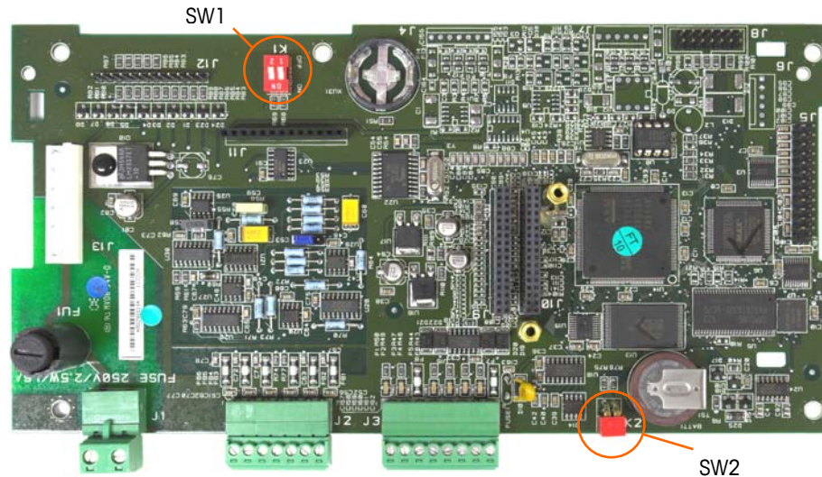
Abbildung 2-49: Hauptplatinenschalter
