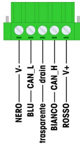
Figura 2-40: Cablaggio al connettore DeviceNet
