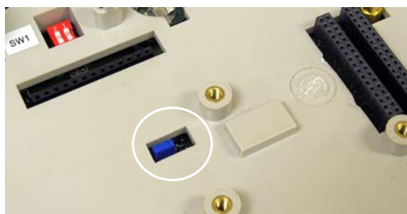
Figura 2-52: Ubicación del puente de milivoltios W1, tapa de PCB principal instalada
