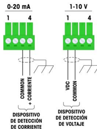
Figura 2-26: Cableado de la salida analógica
