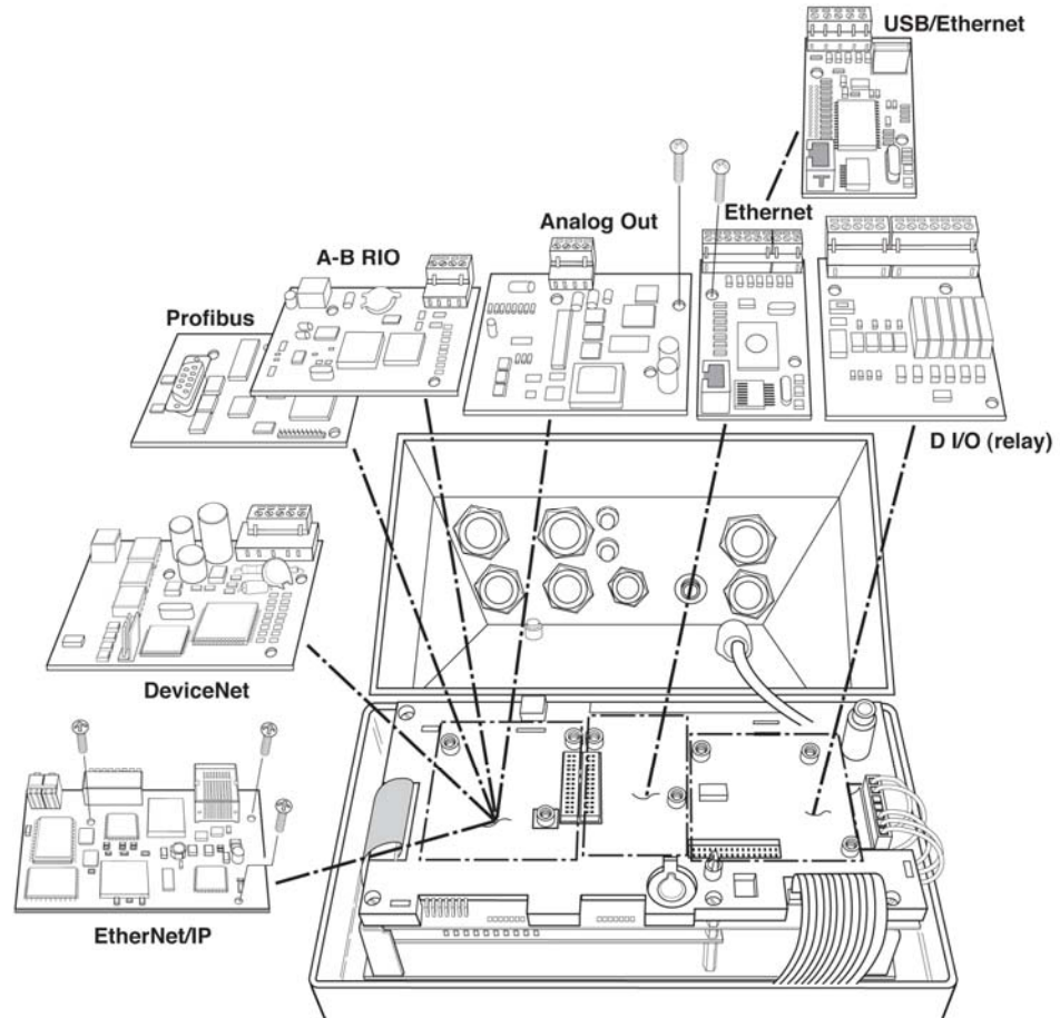
Abbildung 2-23: Positionen der Optionen für das Gehäuse für raue Umgebungen
