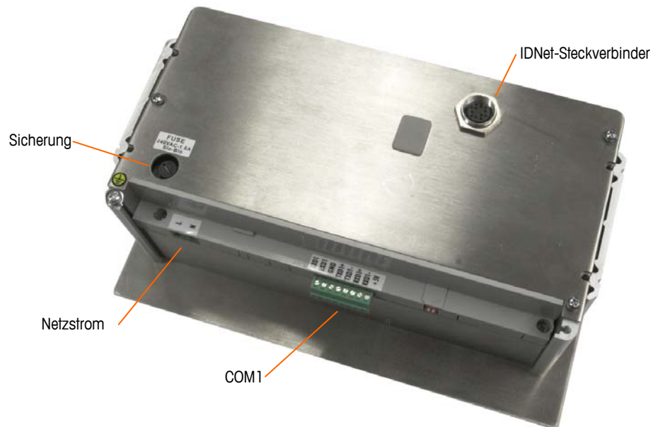
Abbildung 2-16: IDNet-Version im Gehäuse für den Schaltschrankbau
