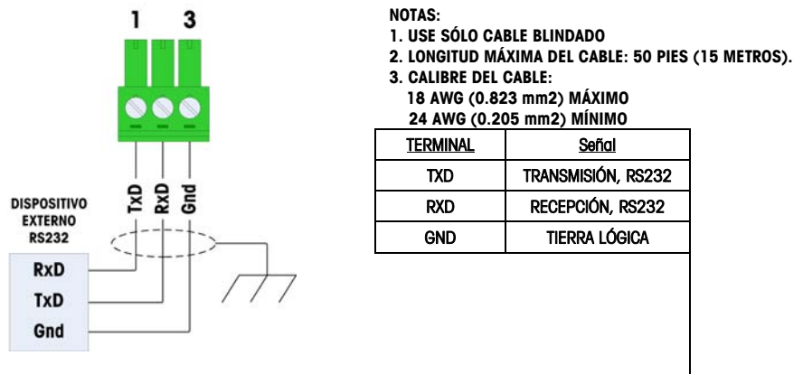
Figura 2-28: Cableado hacia el COM2
