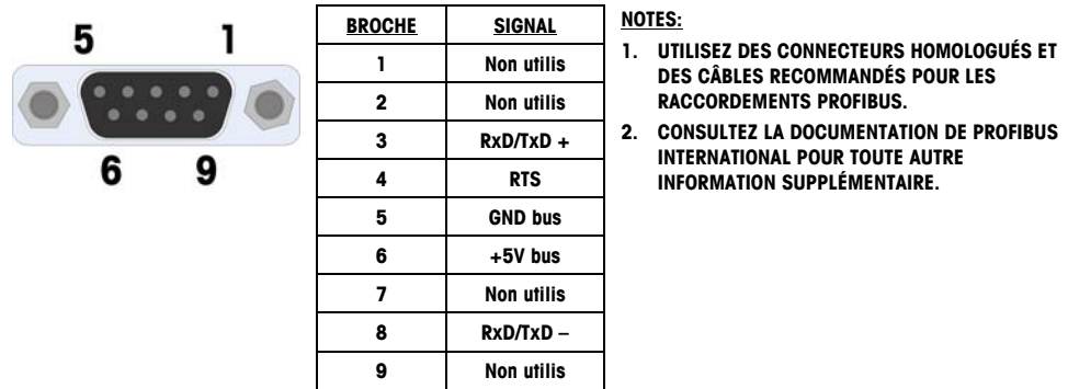
Figure 2-44: Affectations du connecteur PROFIBUS à neuf broches
