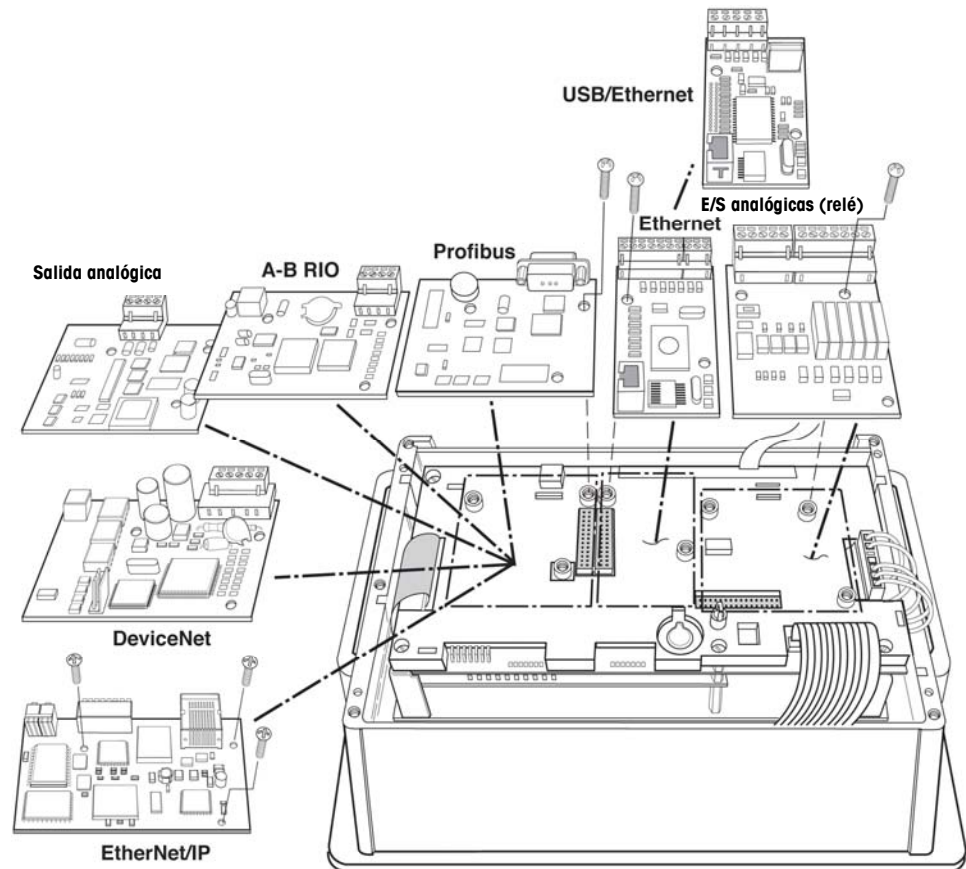
Figura 2-24: Ubicación de las opciones en la caja de montaje en panel
