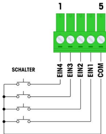
Abbildung 2-33: Aktive Eingangsanschlüsse
