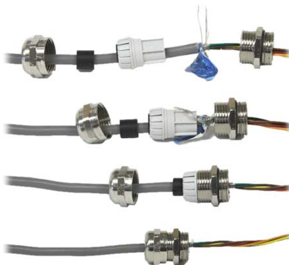
Figure 2-14 : Mise à la terre du blindage du câble
