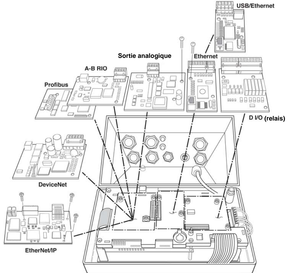
Figure 2-23 : Emplacements des options pour enceinte version environnement hostile
