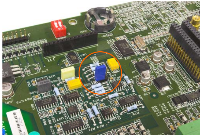
Figure 2-51 : Emplacement du cavalier Millivolt W1, carte principale sans couvercle
