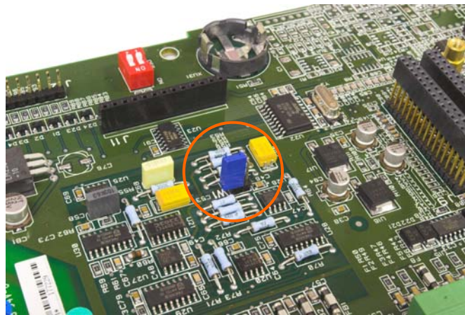
Figura 2-51: Posizione del ponticello Millivolt W1, PCB principale scoperto
