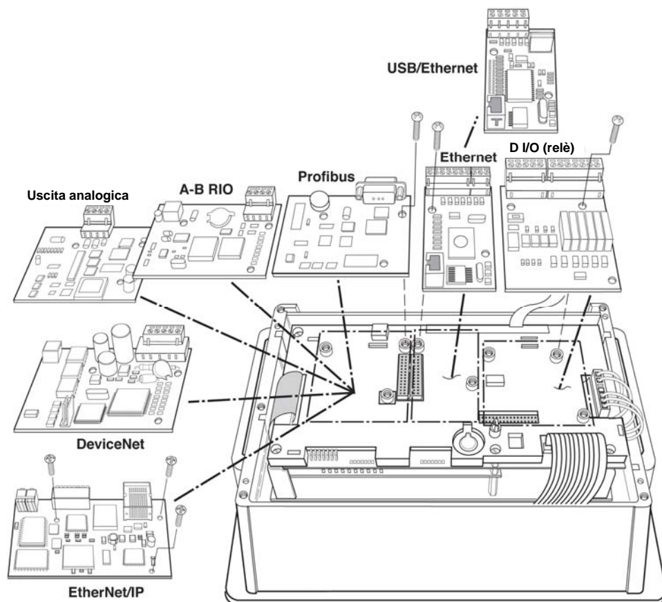
Figura 2-24: Posizione opzioni involucro di montaggio a pannello
