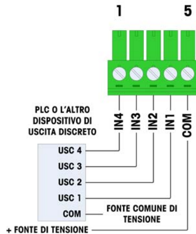
Figura 2-34: Connessioni dell'ingresso passivo
