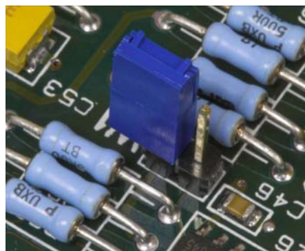
Abbildung 2-53: Einstellungen der W1-Millivolt-Drahtbrücke: Offen / Geschlossen
