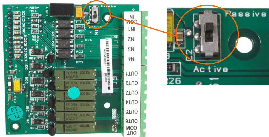
Figura 2-50: Ubicación (i) y configuraciones de interruptor (d) para el interruptor de E/S discontinuas de relé
