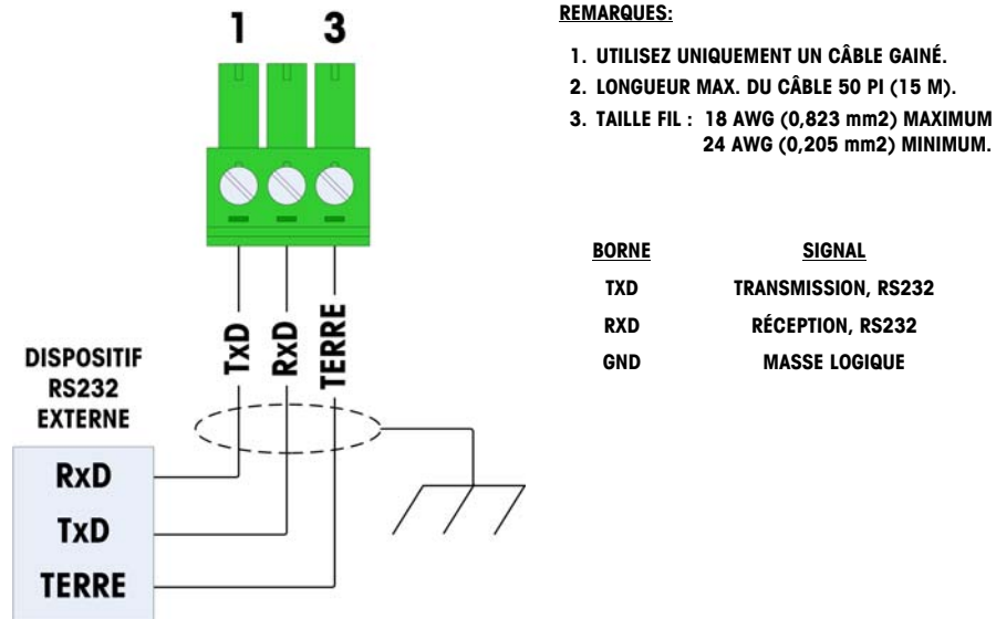
Figure 2-28 : Câblage vers COM2
