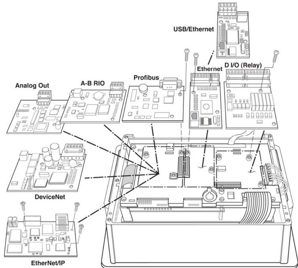
Abbildung 2-24: Positionen der Optionen für das Gehäuse für den Schalttafeleinbau
