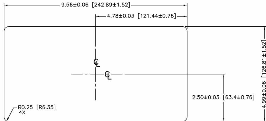
Figura 2-6: Dimensiones del recorte del panel
