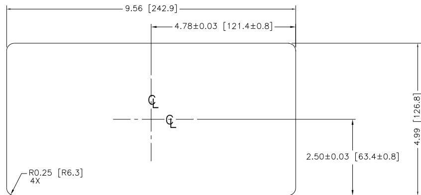
Abbildung 1-3: Abmessungen des Ausschnitts für das IND560-Gehäuse für den Schalttafeleinbau
