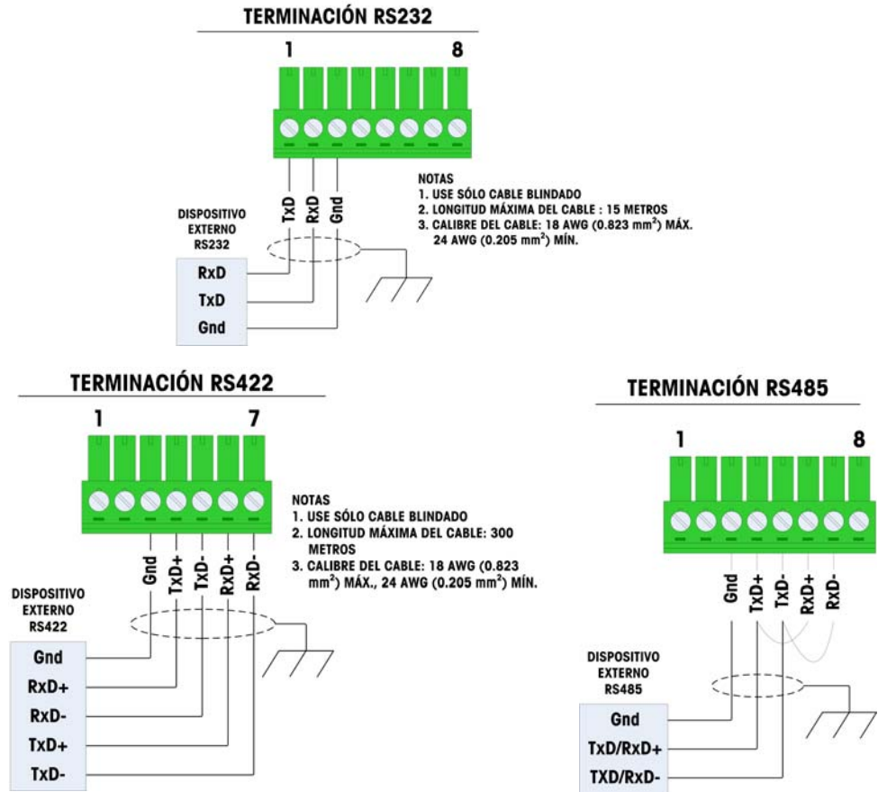
Figura 2-22: Ejemplos de conexiones
