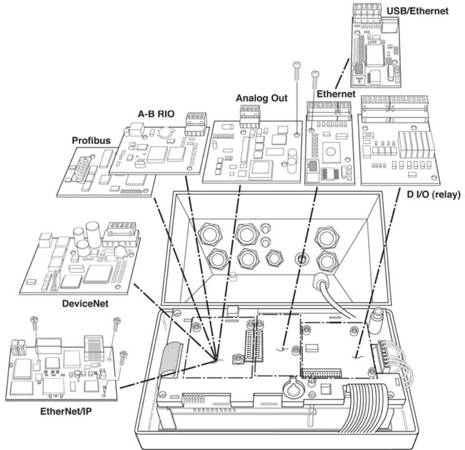
Figura 2-23: Ubicación de las opciones en la caja para ambientes adversos
