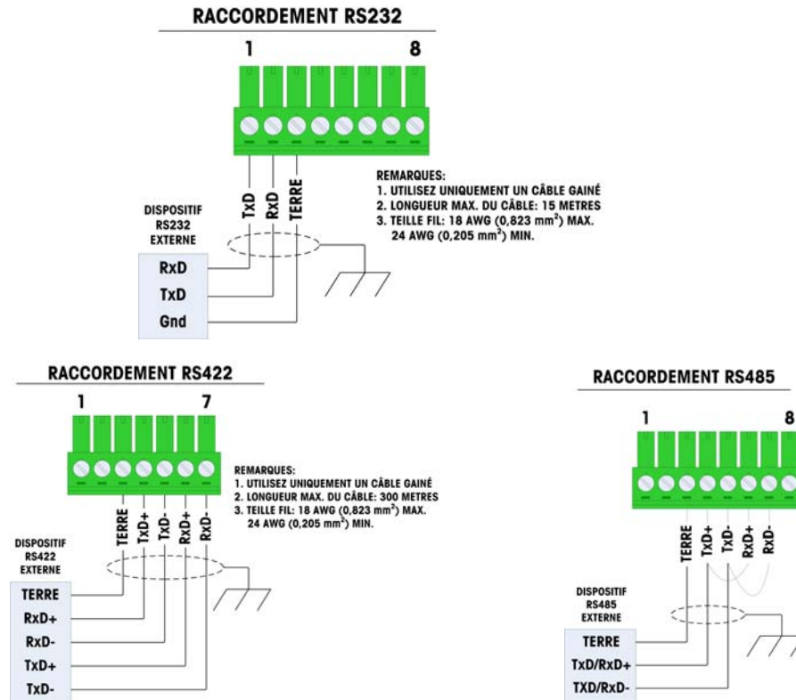
Figure 2-22 : Connexions exemplaires
