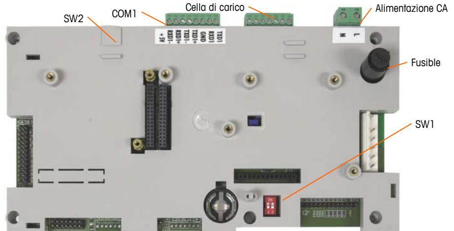
Figura 2-15: Scheda principale analogica in armadietto per ambienti difficili
