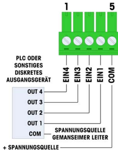
Abbildung 2-34: Passive Eingangsanschlüsse
