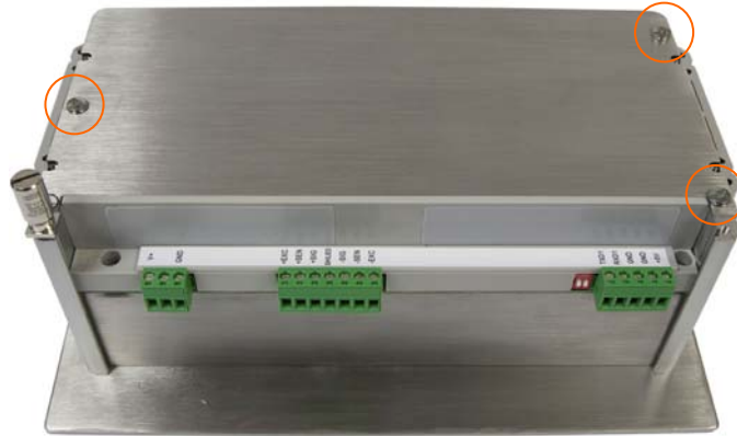
Figura 2-1: Apertura de la caja para montar en panel
