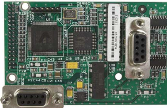
Abbildung 2-41: PROFIBUS-Option für raue Umgebungen
