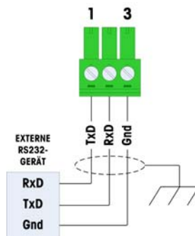
Abbildung 2-28: Verdrahtung mit COM2
