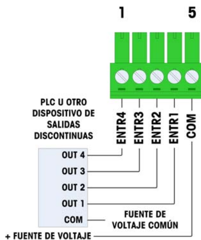
Figura 2-34: Conexiones de entradas pasivas
