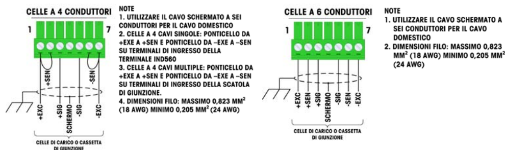
Figura 2-17: Terminazione cella di carico
