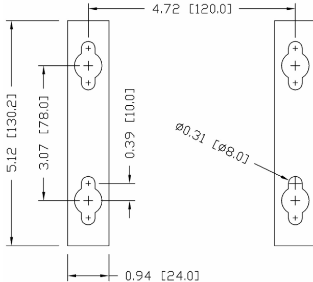
Figura 2-11: Dibujo del patrón de orificios
