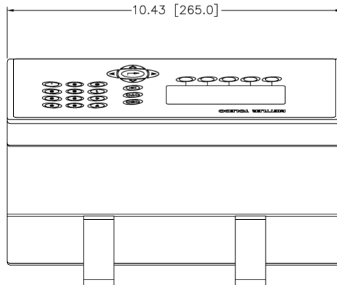
Figura 1-4: Dimensiones de la caja de montaje para ambientes adversos, escritorio o pared del IND560
