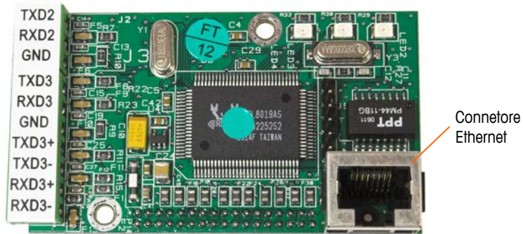
Figura 2-27: Scheda opzionale connessione Ethernet
