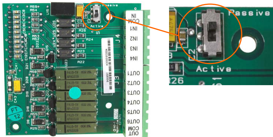
Abbildung 2-50: Position (l) und Schaltereinstellungen (r) für den diskreten I/O-Relaiszugangsschalter
