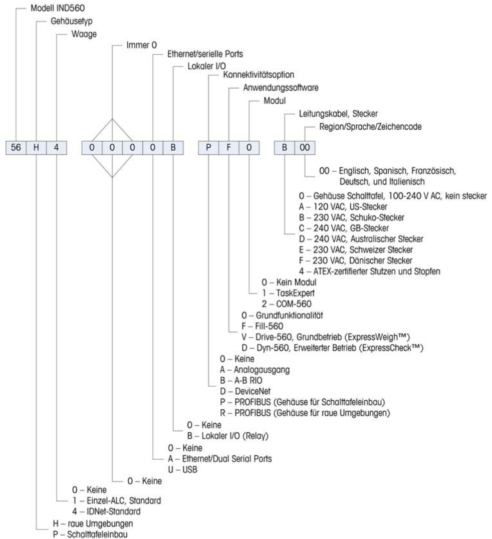
Abbildung 1-1: IND560-Modellidentifikationsnummern
