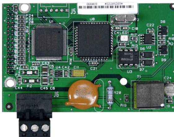
Figura 2-36: Opción RIO
