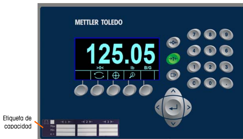
Figura 2-55: Instalación de la etiqueta
