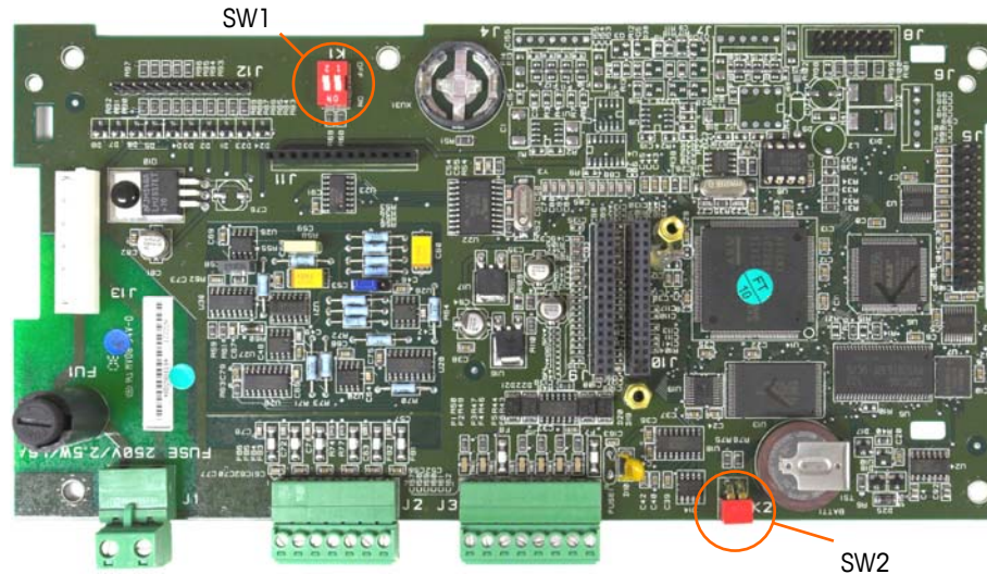
Figure 2-49: Commutateurs de la carte PCB principale
