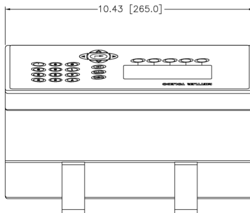
Abbildung 1-4: Abmessungen des IND560-Modells für raue Umgebungen und Tisch-/Wandmontage
