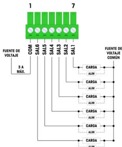
Figura 2-35: Salidas de relé
