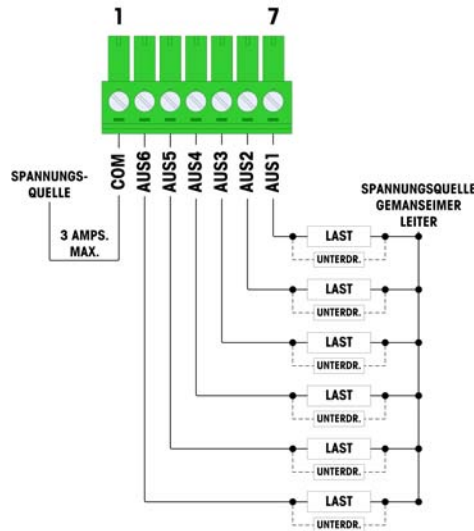
Abbildung 2-35: Relaisausgänge
