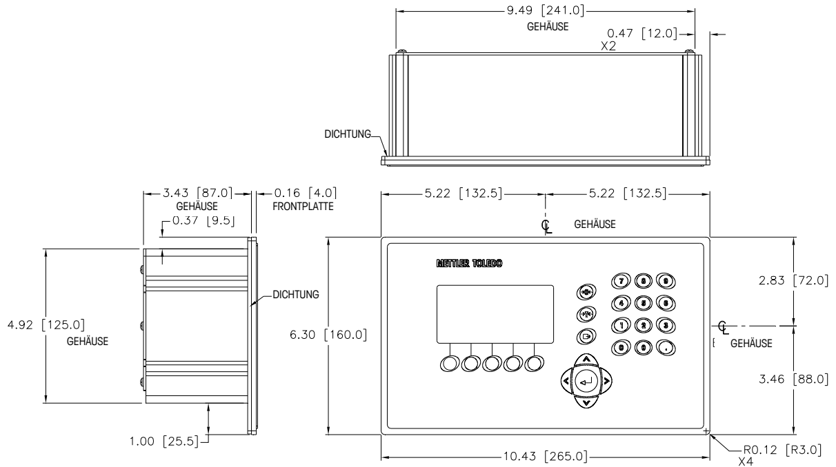
Abbildung 1-2: Abmessungen des IND560-Gehäuses für den Schalttafeleinbau
