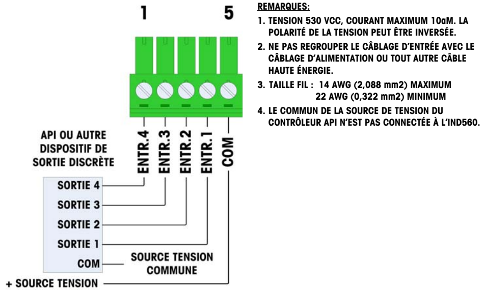
Figure 2-34 : Connexions vers entrée passive
