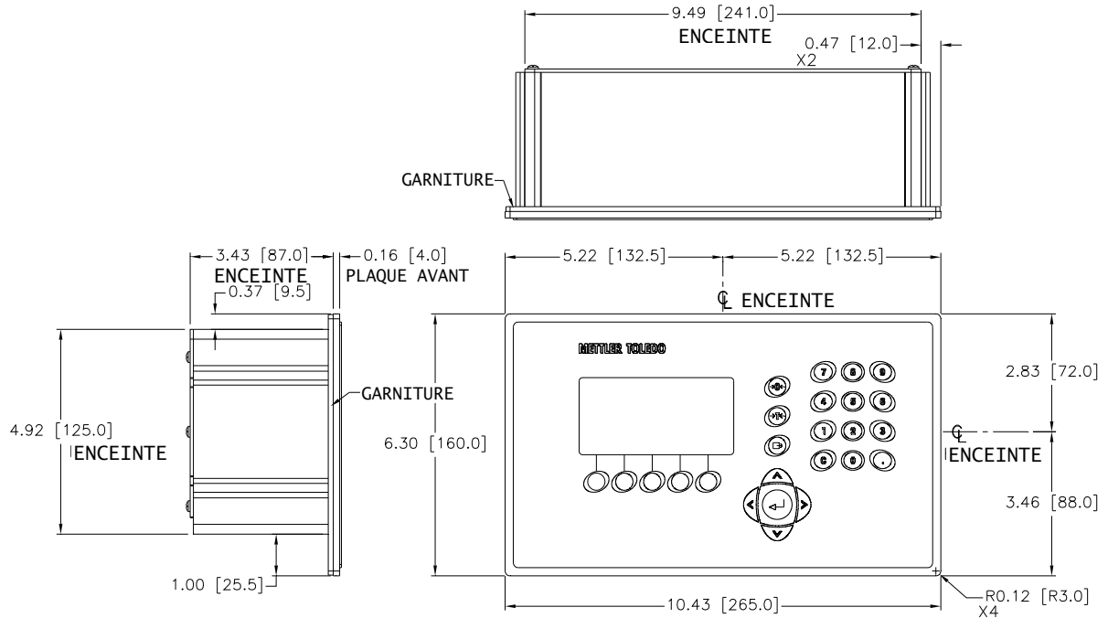
Figure 1-2 : Dimensions pour l'enceinte de montage sur tableau de l'IND560
