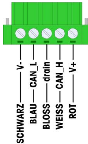
Abbildung 2-40: DeviceNet-Anschlussverdrahtung
