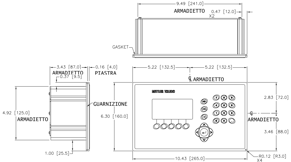
Figura 1-2: Dimensioni del montaggio a pannello dell'IND560
