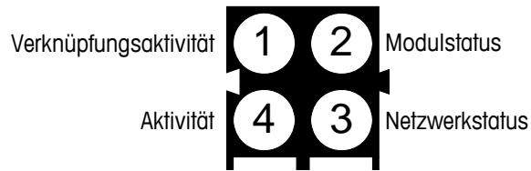
Abbildung 2-46: Statusanzeiger-LEDs für Ethernet / IP
