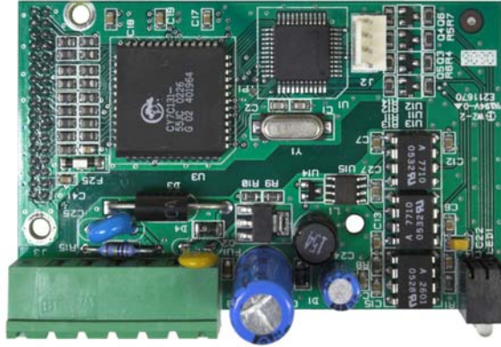
Figura 2-38: Scheda opzionale DeviceNet
