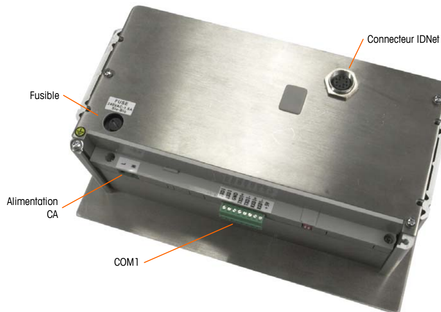
Figure 2-16 : Version IDNet dans enceinte avec montage sur tableau
