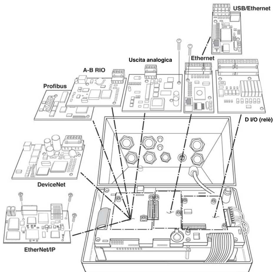
Figura 2-23: Posizione opzioni involucro rigido
