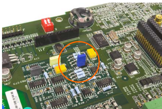
Figura 2-51: Ubicación del puente de milivoltios W1, PCB principal descubierta
