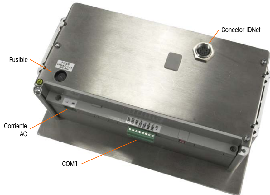
Figura 2-16: Versión IDNet en caja de montaje en panel
