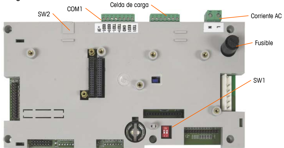
Figura 2-15: Tablero principal analógico en caja para ambientes adversos
