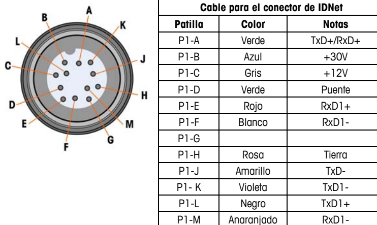
Figura 2-20: Asignaciones de las patillas del conector de IDNet
