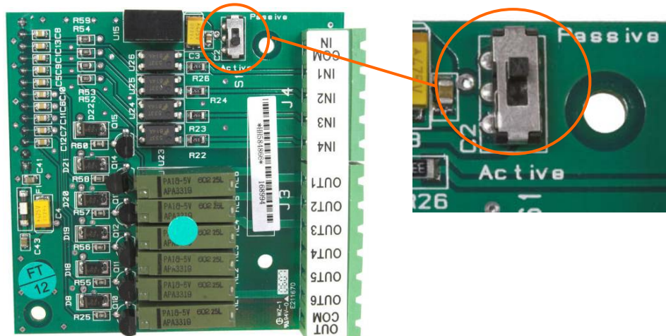
Figura 2-50: Posizione (s) e impostazioni dell'interruttore (d) per l'interruttore di ingresso I/O discreto del relè
