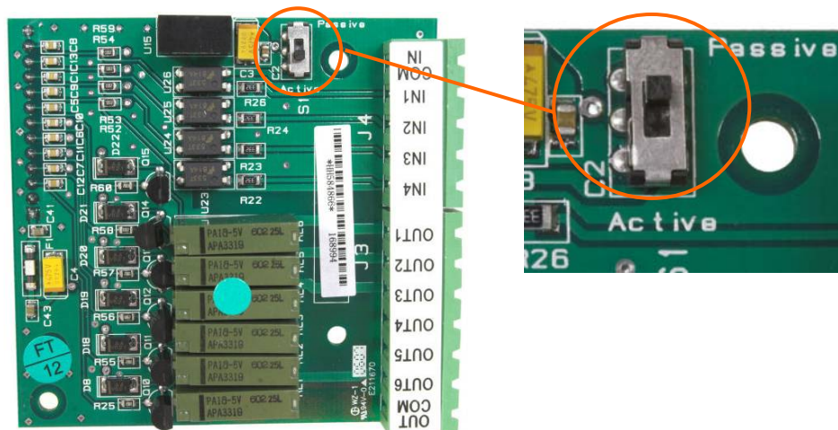
Figure 2-50 : Emplacement (g) et réglages du commutateur (d) pour le commutateur d'entrée E/S discrètes relais
