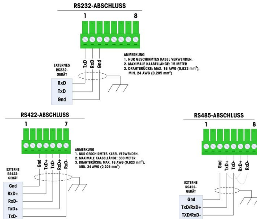
Abbildung 2-22: Anschlussbeispiele
