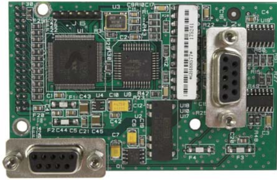
Figura 2-41: Opción PROFIBUS hacia la caja para ambientes adversos
