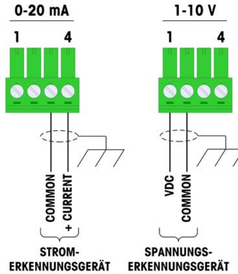
Abbildung 2-26: Verdrahtung des Analogausgangs
