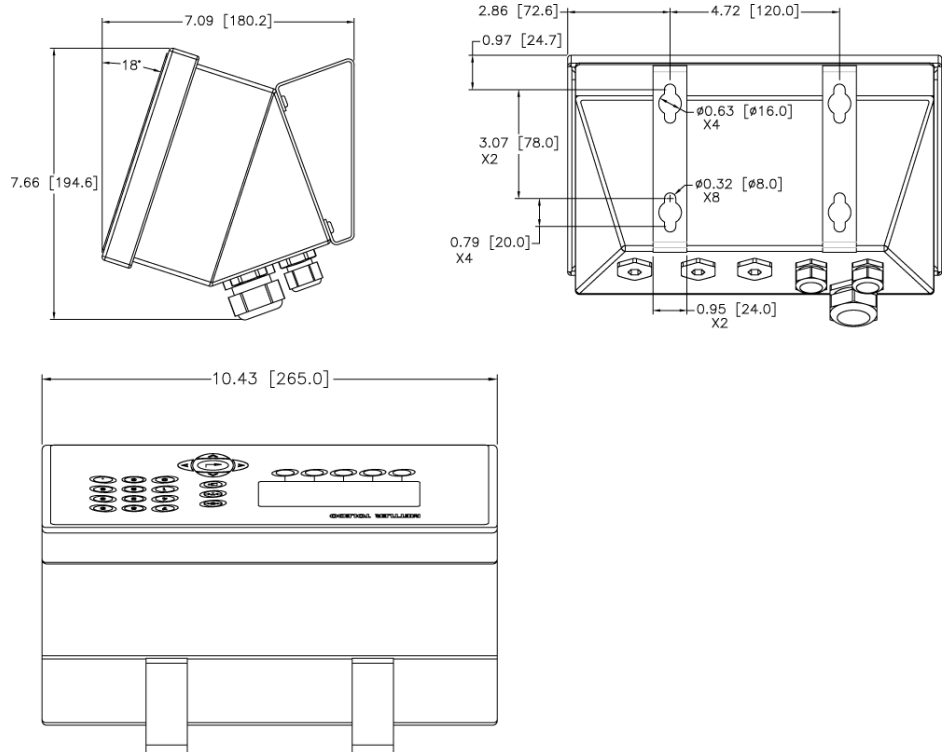
Figura 1-5: Dimensioni dell'involucro rigido del terminale IND560 per montaggio a parete, con staffe opzionali
