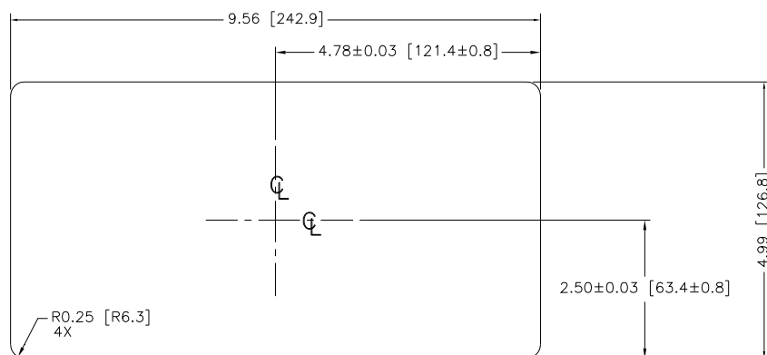
Figura 1-3: Dimensiones del recorte para montaje en panel del IND560
