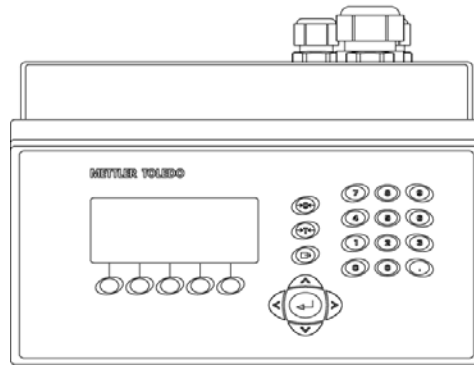
Figura 1-4: Dimensioni dell'involucro rigido del terminale IND560 per montaggio a banco
