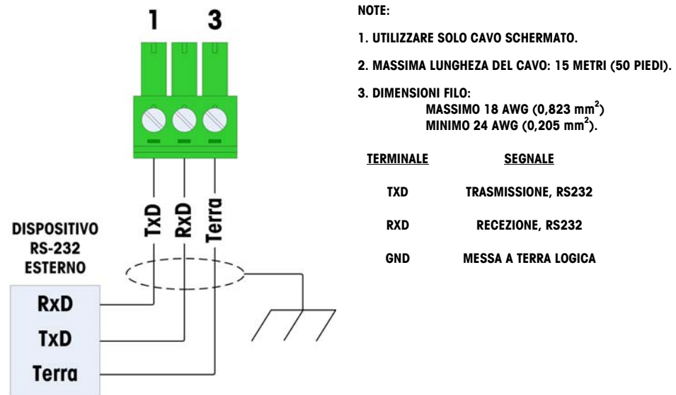
Figura 2-28: Cablaggio COM2
