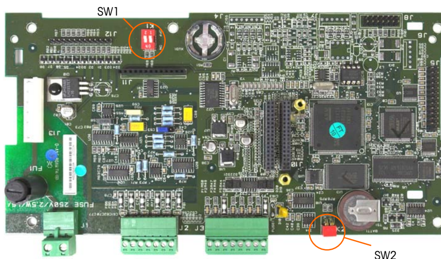
Figura 2-49: Interruttori del PCB principale
