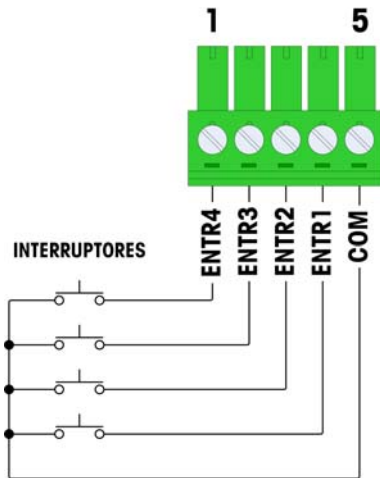
Figura 2-33: Conexiones de entradas activas
