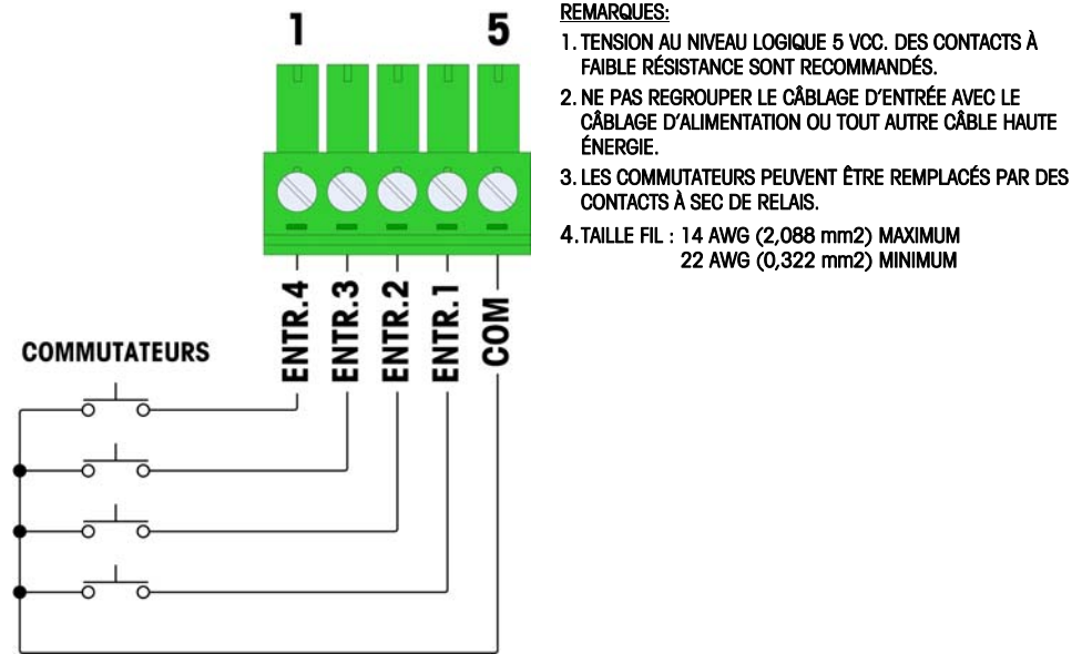
Figure 2-33 : Connexions vers une entrée active
