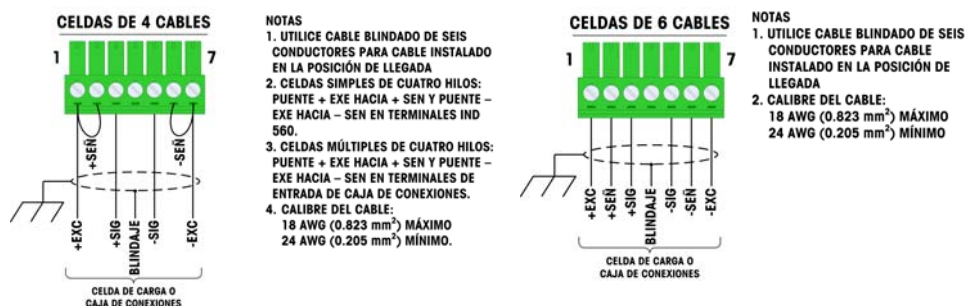
Figura 2-17: Terminación de las celdas de carga
