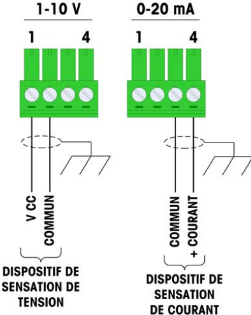
Figure 2-26 : Câblage de la Sortie analogique
