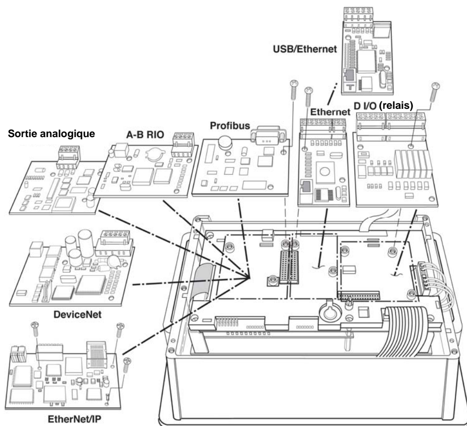
Figure 2-24 : Emplacements des options pour enceinte version montage sur tableau
