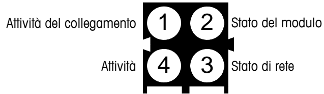
Figura 2-46: LED degli indicatori di stato EtherNet / IP
