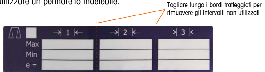
Figura 2-54: Preparazione dell'etichetta di capacità
