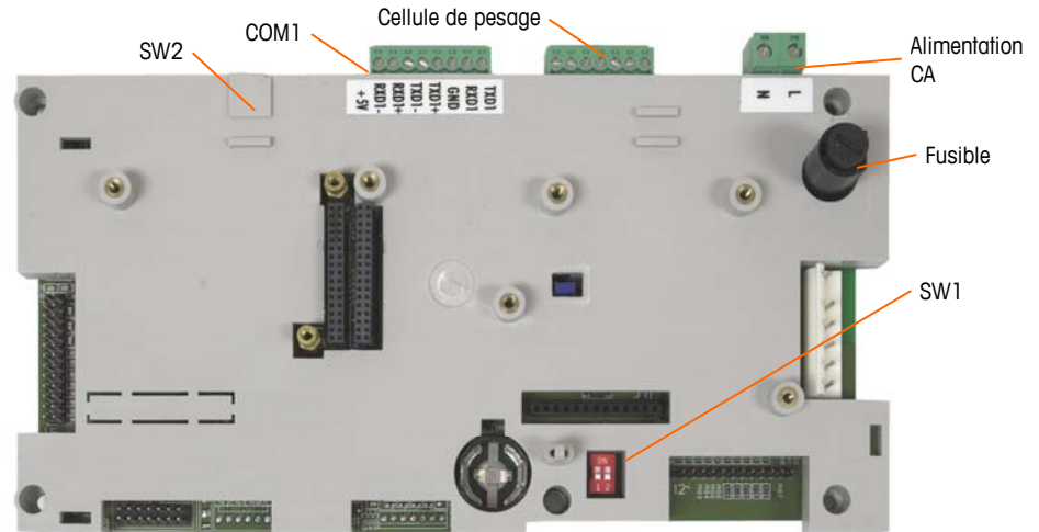
Figure 2-15 : Carte principale analogique dans une enceinte pour environnement hostile
