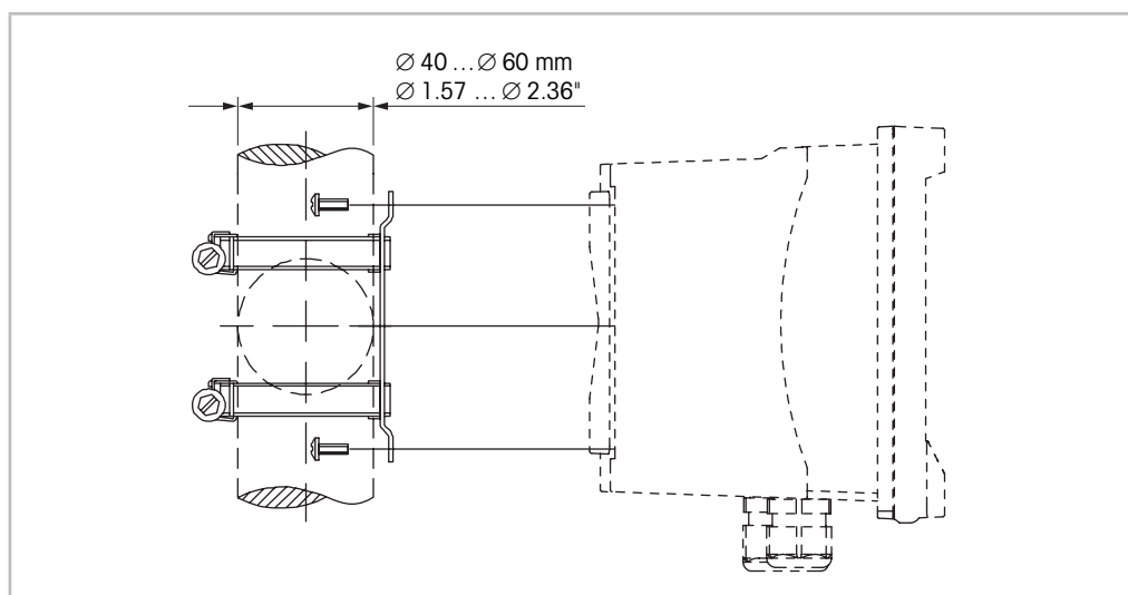
図 8: 配管取り付け½DINバージョン
