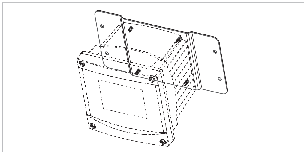
図 7: 壁設置 (壁設置キット)
