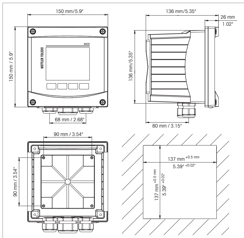
図 4: 寸法 \frac{1}{2} DINバージョン
