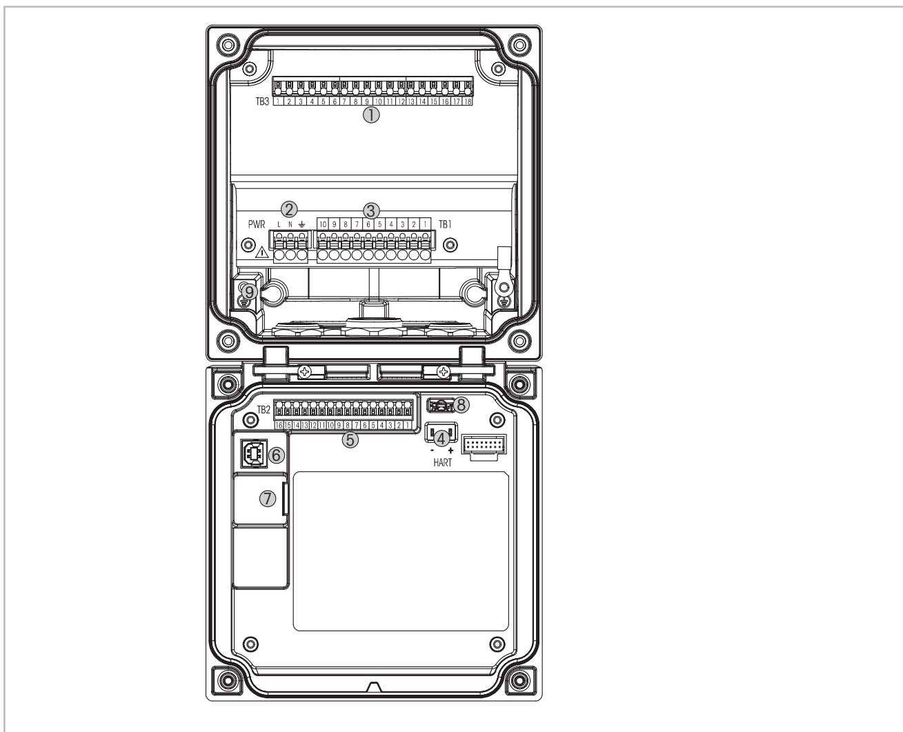
図 9: M400 1/2 DINバージョン
