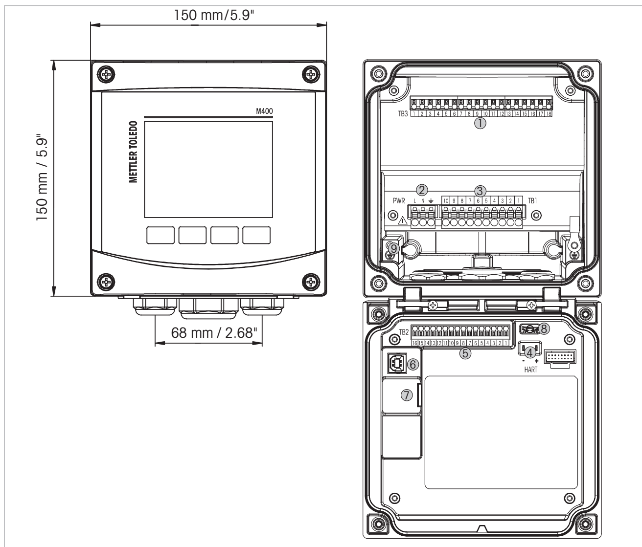
図 1: M400 ½DINバージョン
