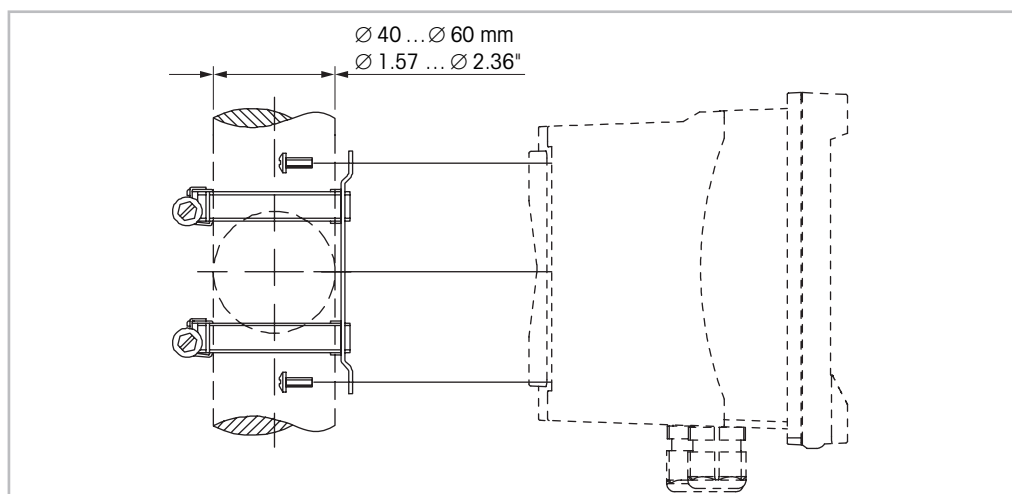
图8: ½ DIN 型号的管道安装
