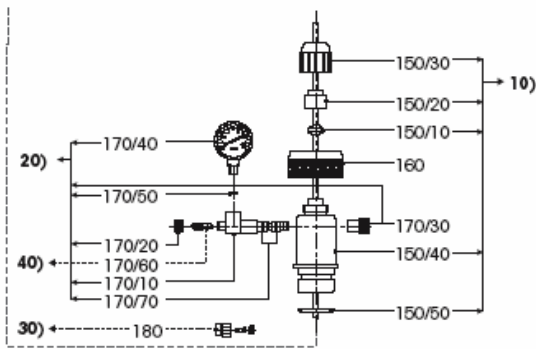
Top piece / Oberteil / Tête InFit 763 e
