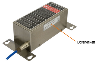
Abbildung 1-2: Position des Akkupack-Datenetiketts
