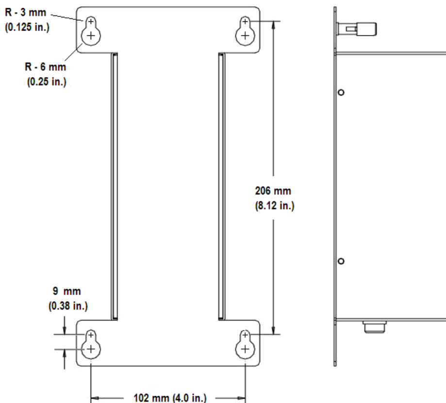
Figura 3-2: Dimensioni Montaggio batteria
