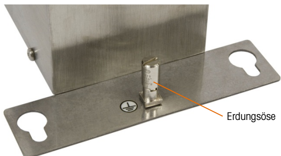
Abbildung 3-6: Erdung
