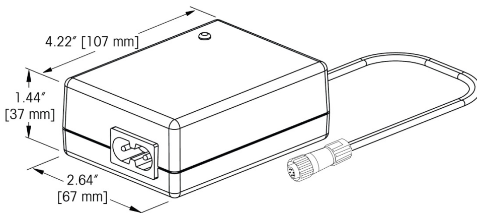
Figura 1-7: dimensões físicas do carregador de bateria
