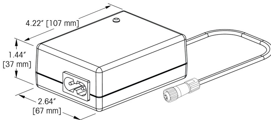
Figura 1-7: Dimensioni fisiche del caricabatteria
