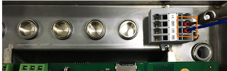
Figura 3-3: Cableado con el conector de la terminal
