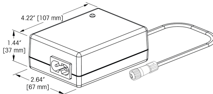
Abbildung 1-7: Abmessungen des Cell-Con Ladegeräts
