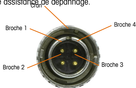
Figure 4-3: Emplacement des broches du connecteur du batterie
