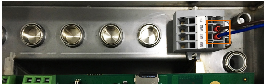
Figura 3-3: Fiação para o conector de terminal
