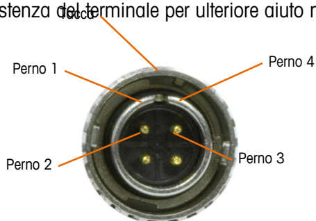
Figura 4-3: Designazioni del pin della batteria
