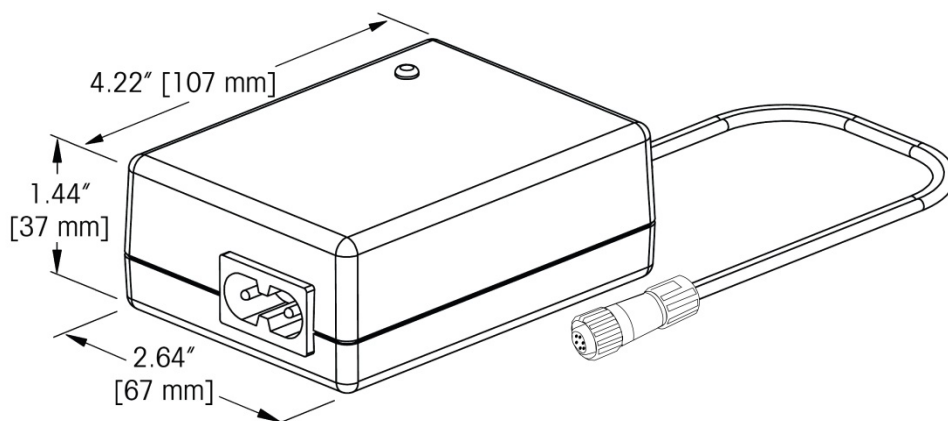
Figure 1-7: Dimensions physiques du chargeur
