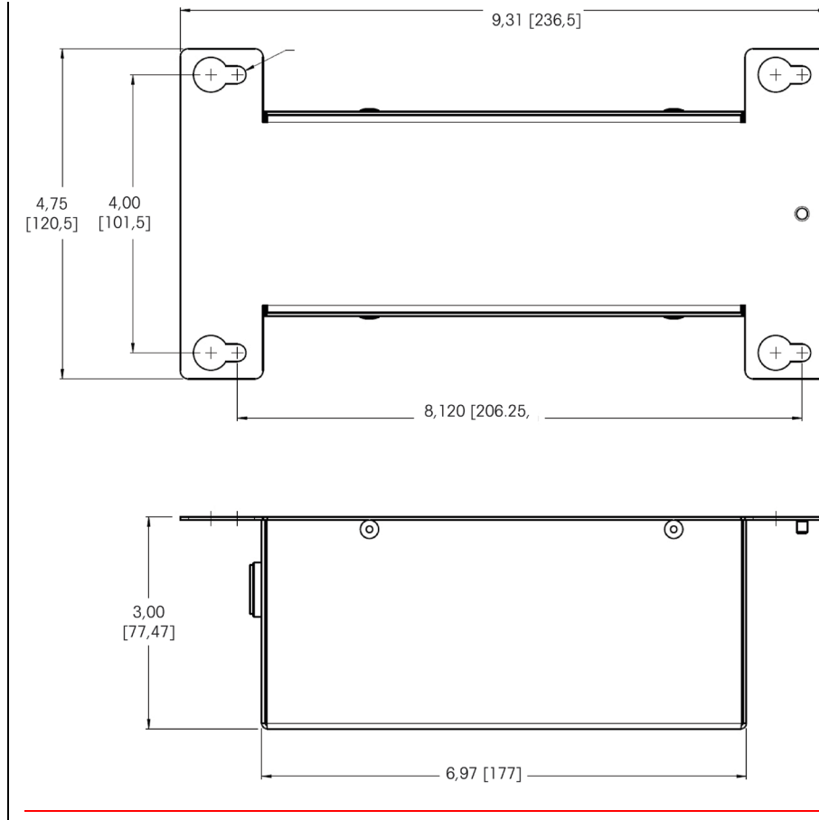
Abbildung 1-5: Allgemeine Abmessungen des Akkupacks 30538111
