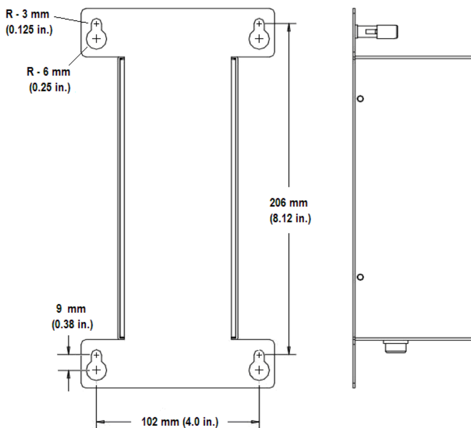
Figure 3-2 : Dimensions de montage de la batterie
