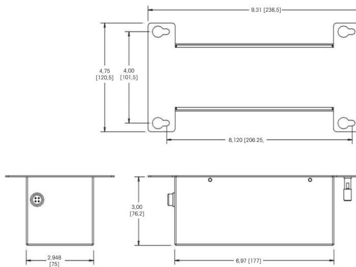
Abbildung 1-4: Allgemeine Abmessungen des Akkupacks 64060625
