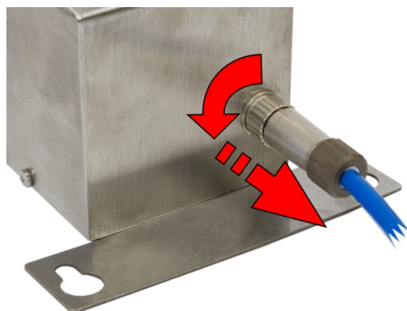
Figure 3-5 : Déconnexion du bloc de batteries
