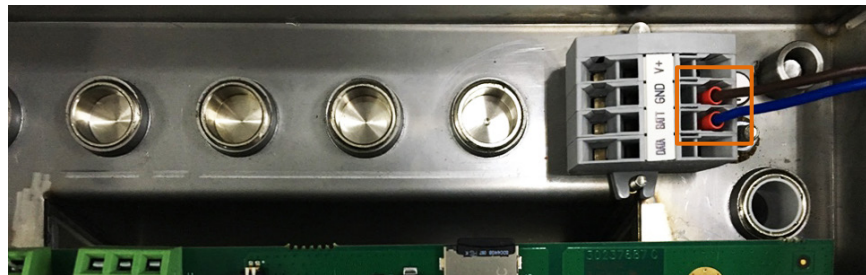
Figura 3-3: Cablaggio al connettore di terminale
