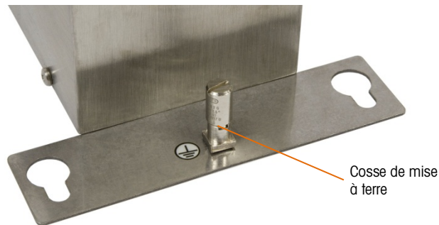
Figure 3-6 : Connexion à la terre
