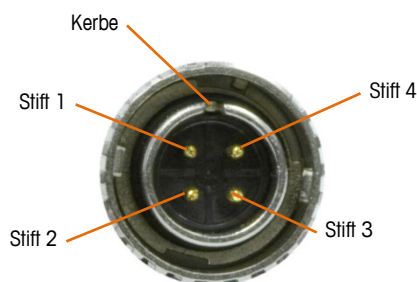
Abbildung 4-3: Stift Definitionen
