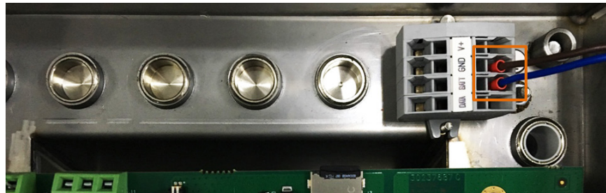
Abbildung 3-3: Verdrahtung zum Terminal-Steckanschluss
