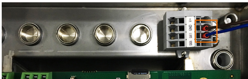
Figure 3-3 : Câblage au connecteur du terminal
