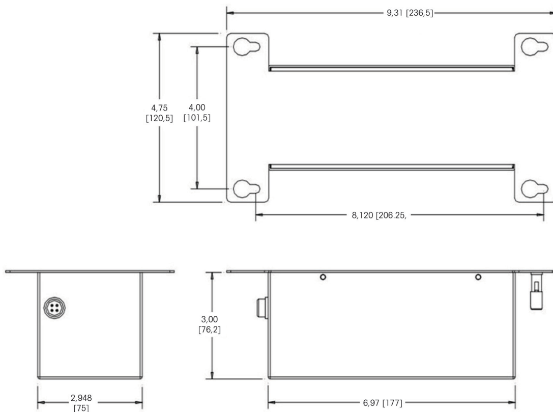
Figura 1-4: Dimensões gerais do pacote de baterias 64060625
